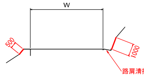
標準断面図 S=1/100
